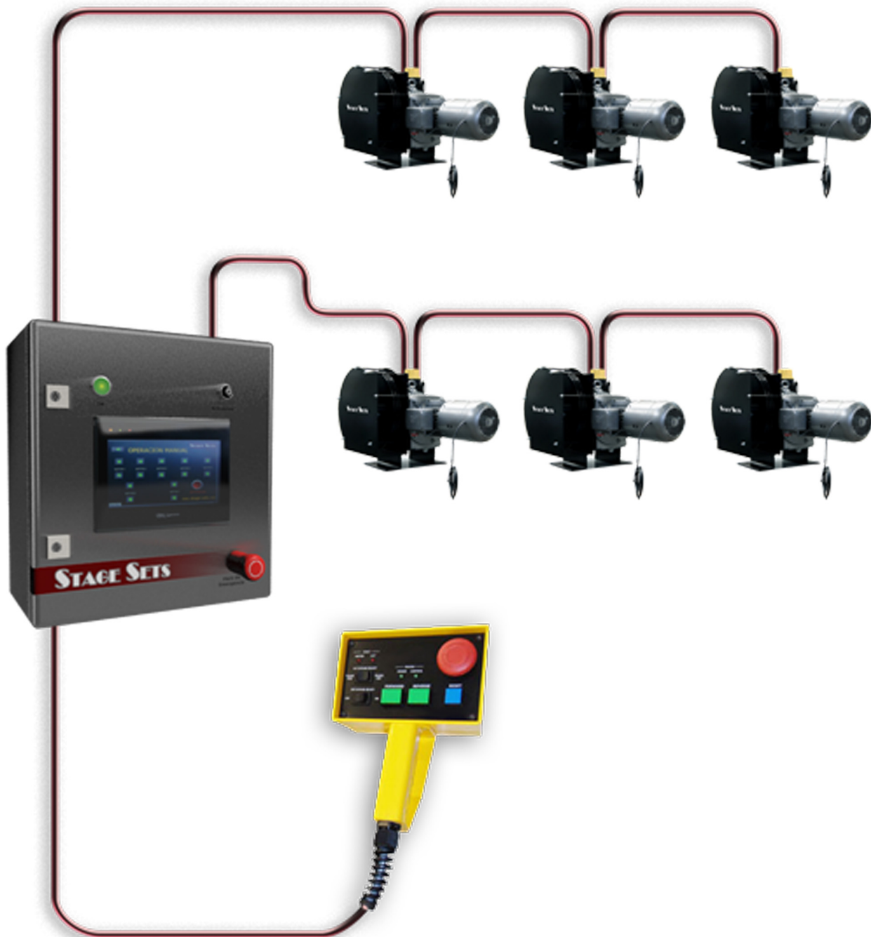
Diagrama de Conexión
